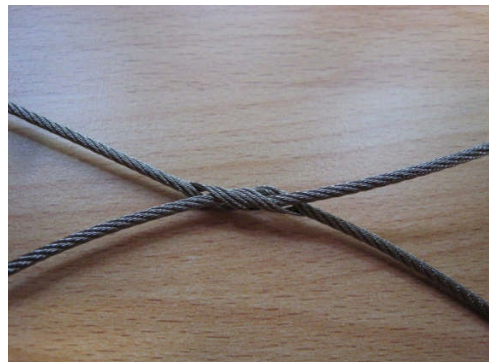
Seilnetze aus rostfreiem Stahl, 60 mm x 60 mm, \Phi 2,0 mm
