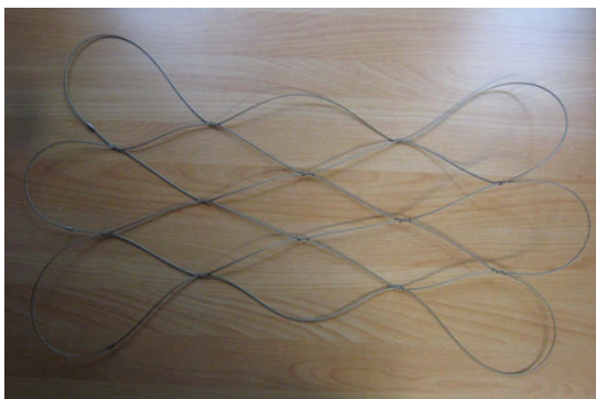
Seilnetze aus rostfreiem Stahl, 60 mm x 60 mm, \Phi 2,0 mm
